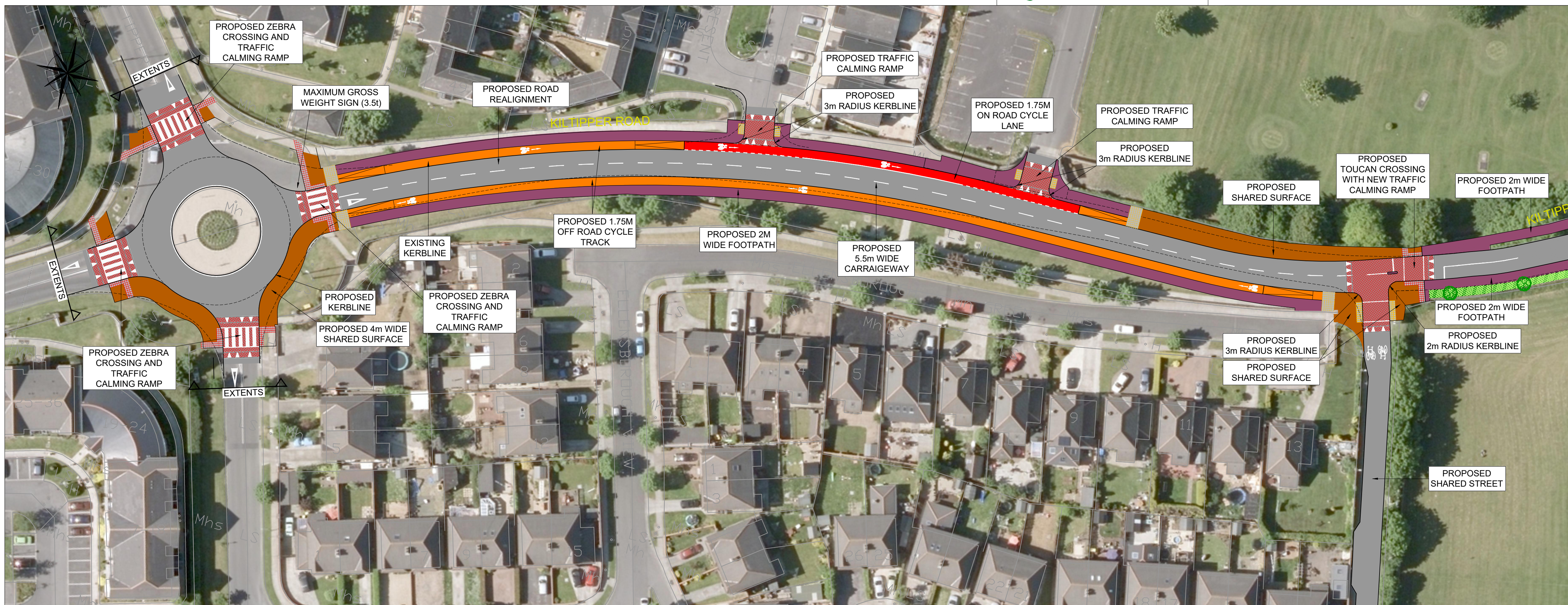
LAYOUT - 6 SCALE: 1:500
