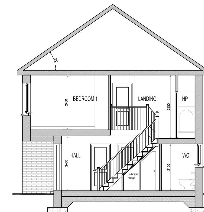
K5 - SECTION A-A
