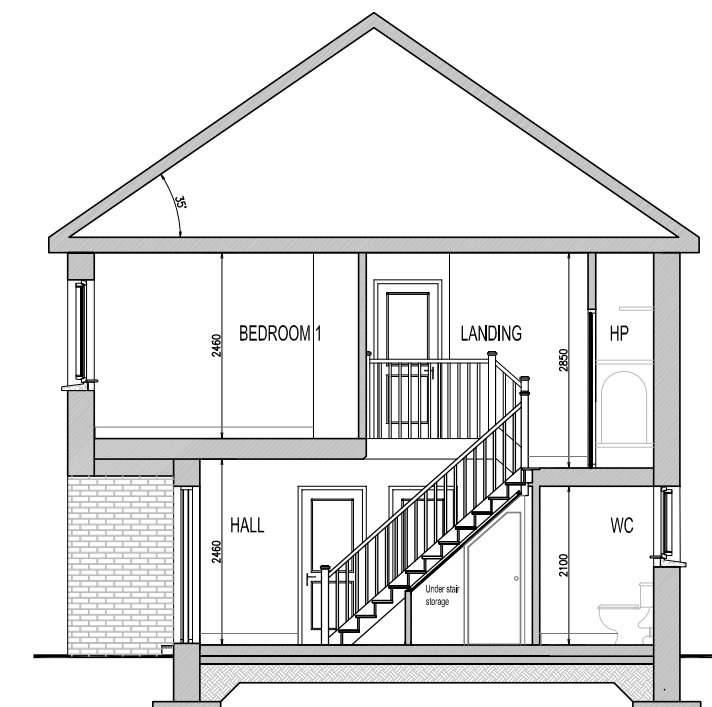
K4 - SECTION A-A
