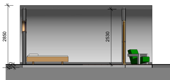
7 POD SECTION 1 1 : 100
