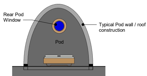
6 POD SECTION 2 1 : 100
