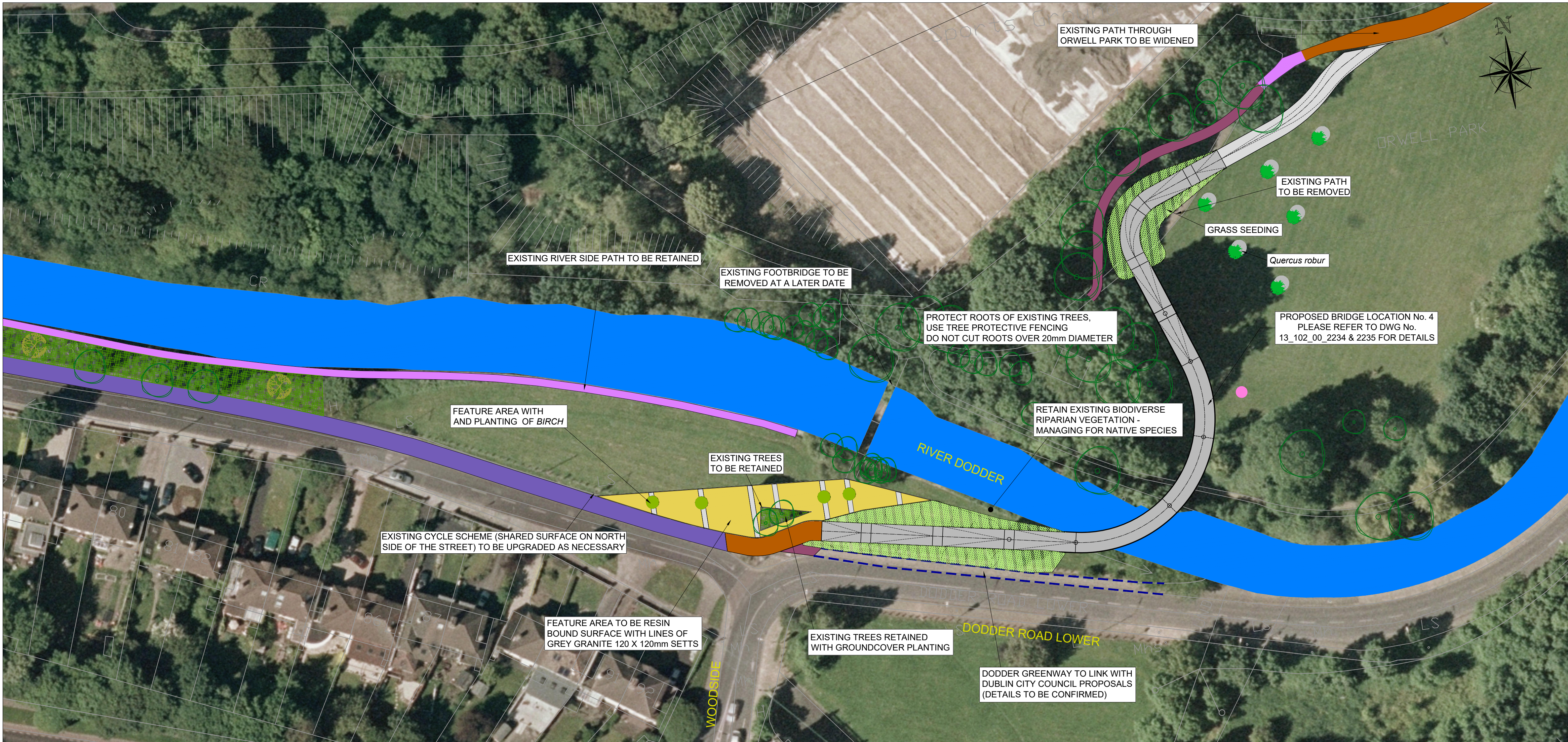
LAYOUT - 43 SCALE: 1:500
