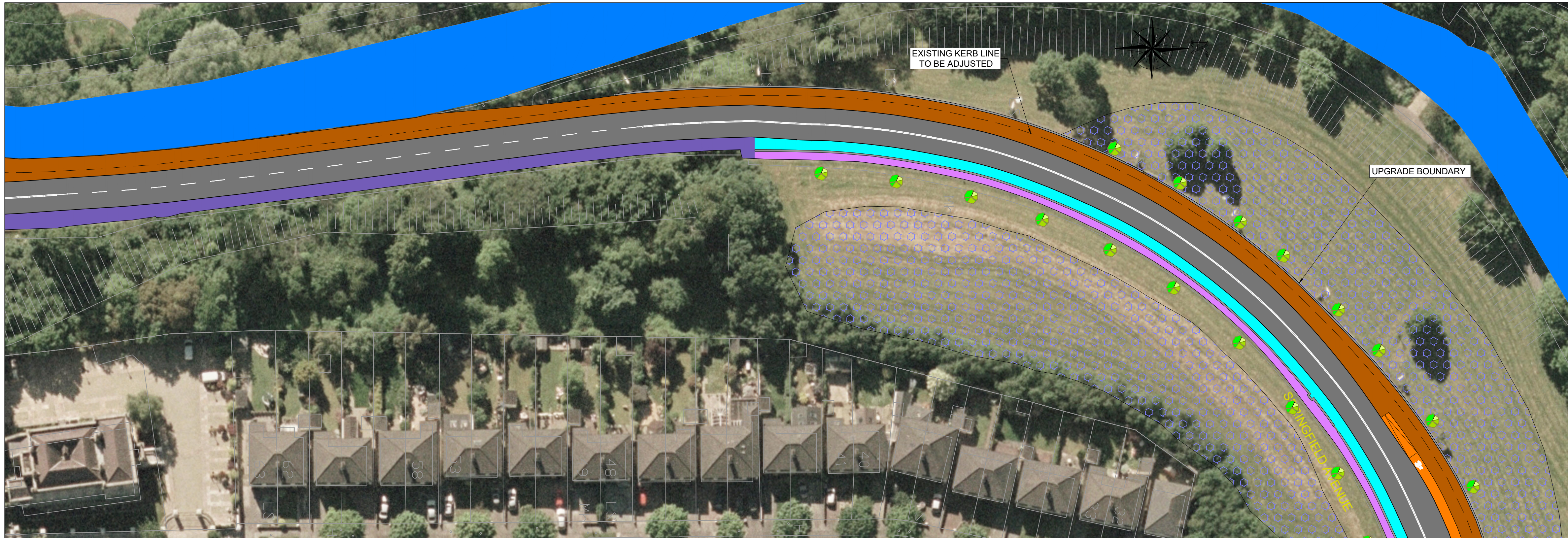
LAYOUT - 39 SCALE: 1:500
