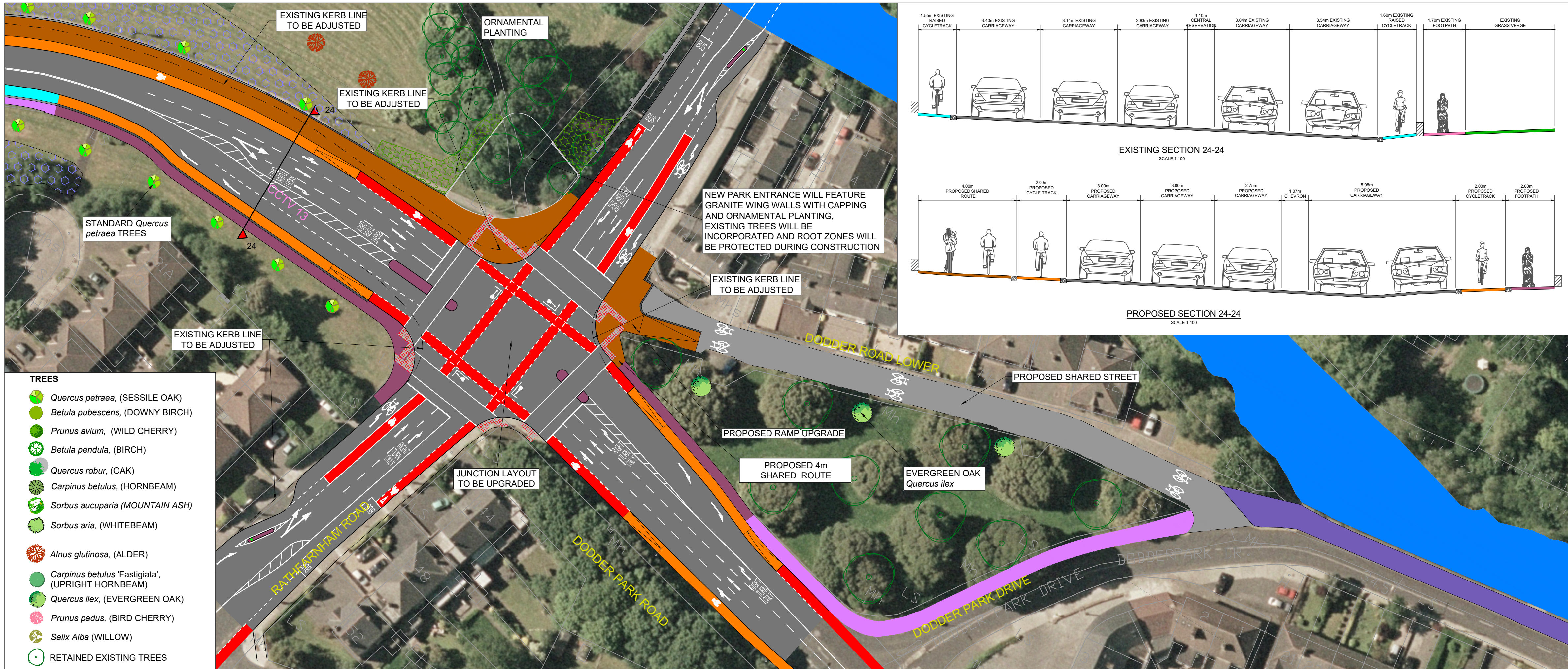
LAYOUT - 40 SCALE: 1:500
