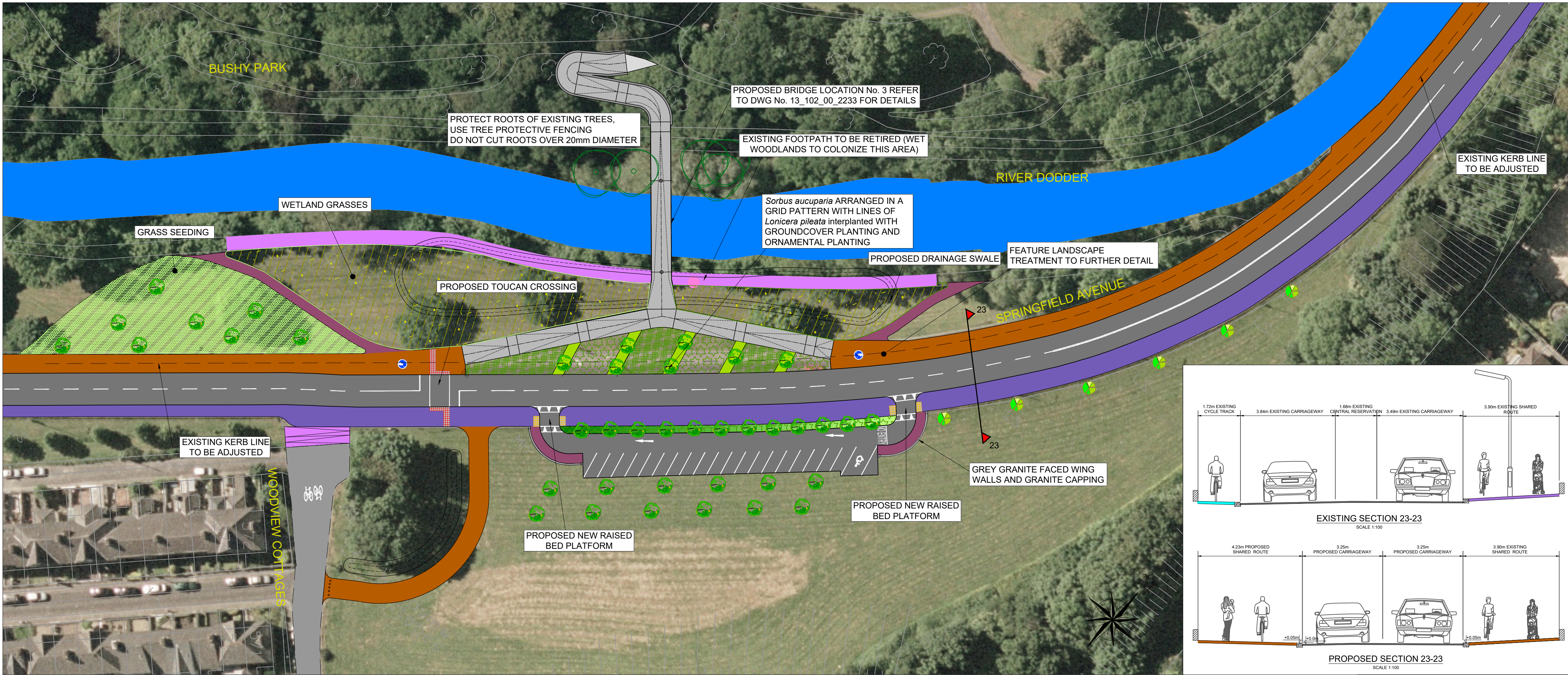
LAYOUT - 37 SCALE: 1:500
