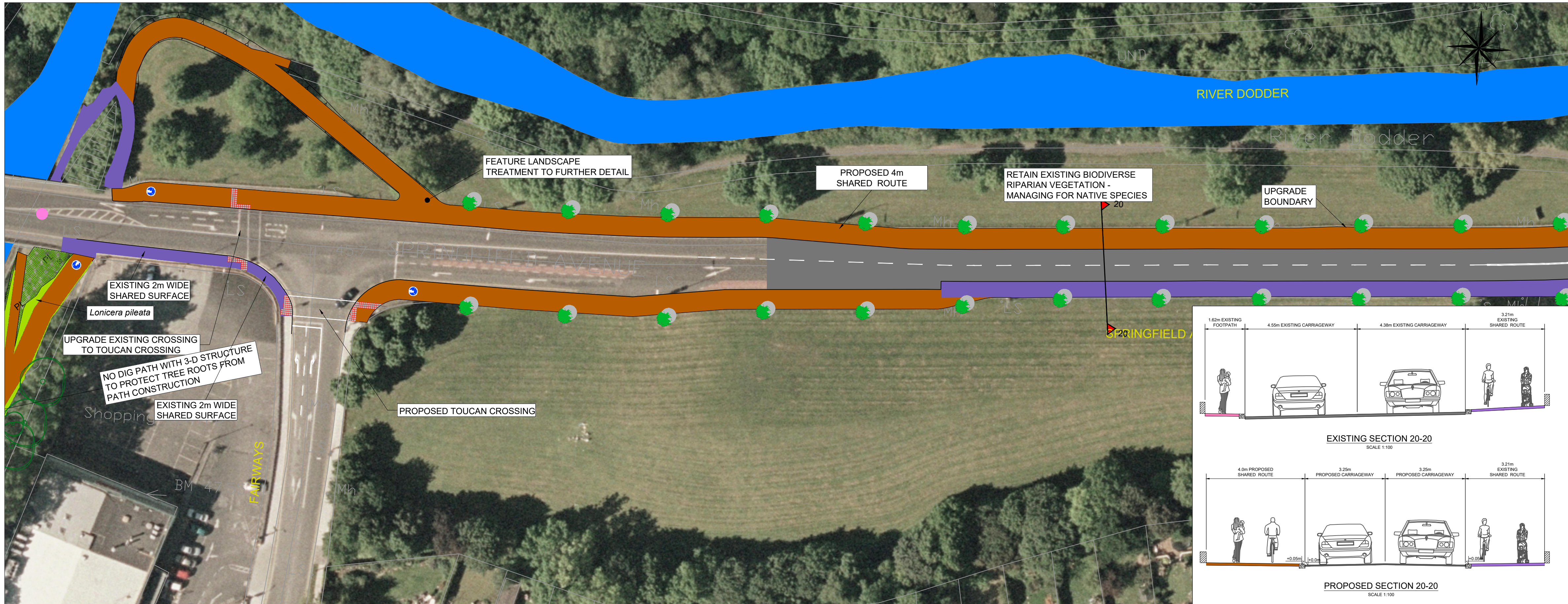
LAYOUT - 35 SCALE: 1:500
