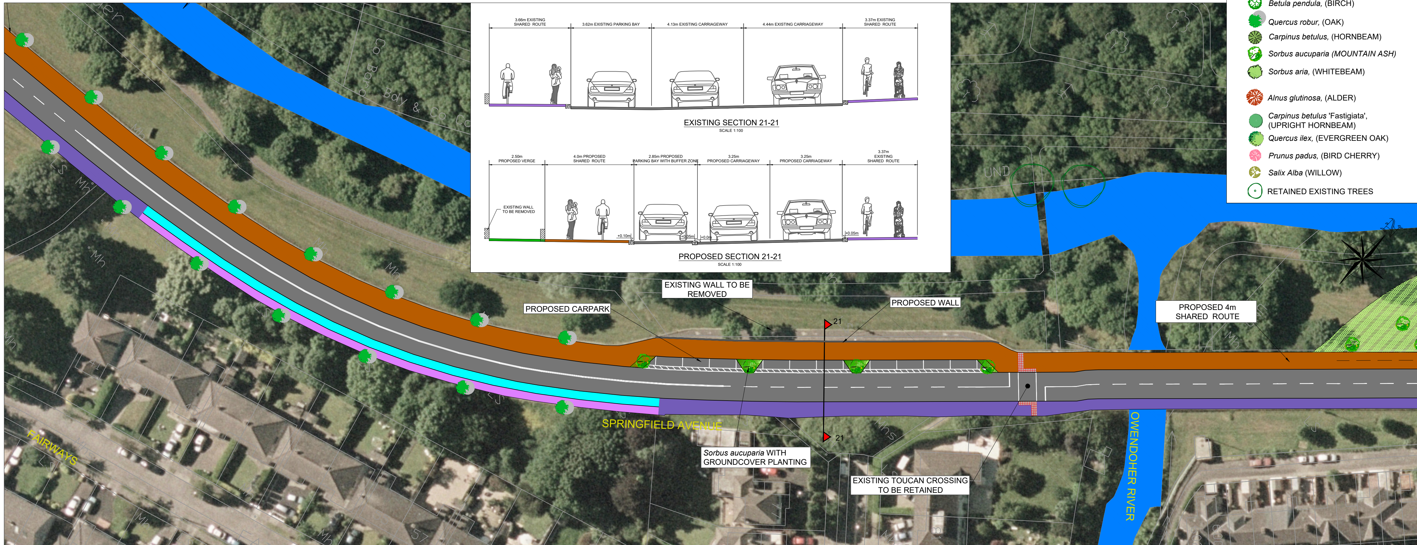
LAYOUT - 36 SCALE: 1:500
