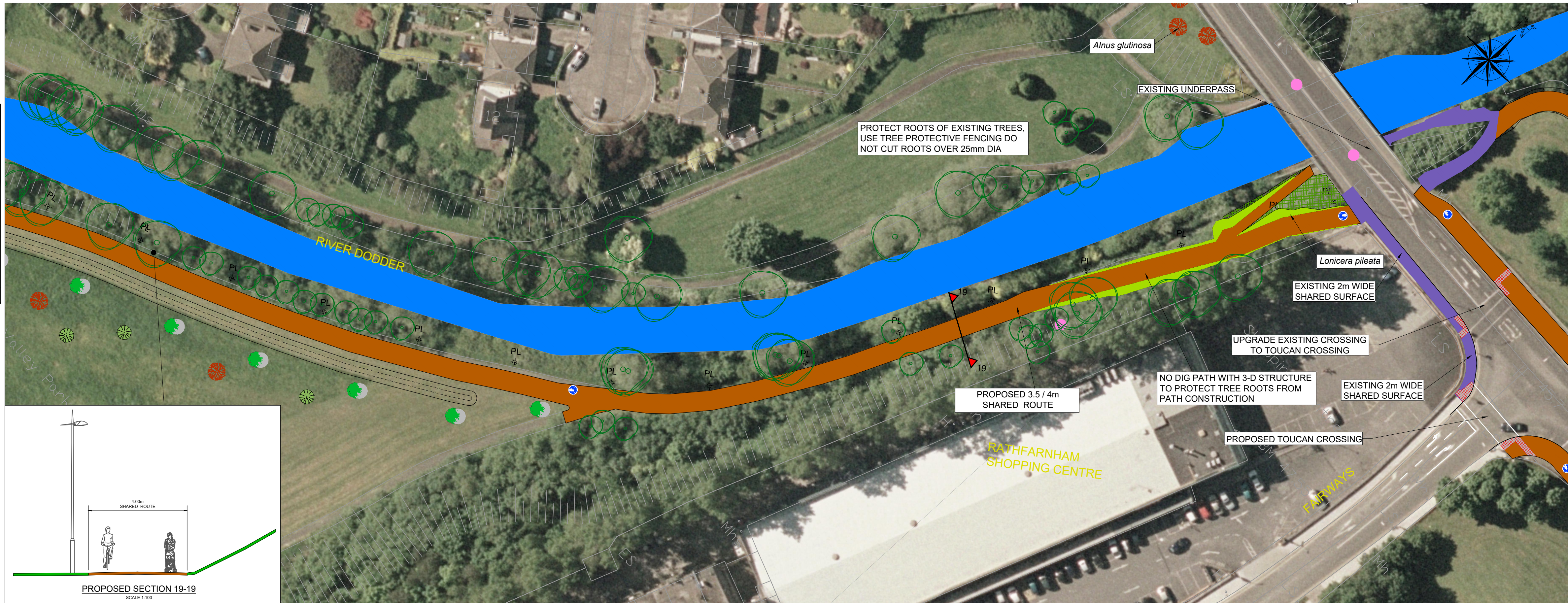
LAYOUT - 34 SCALE: 1:500
