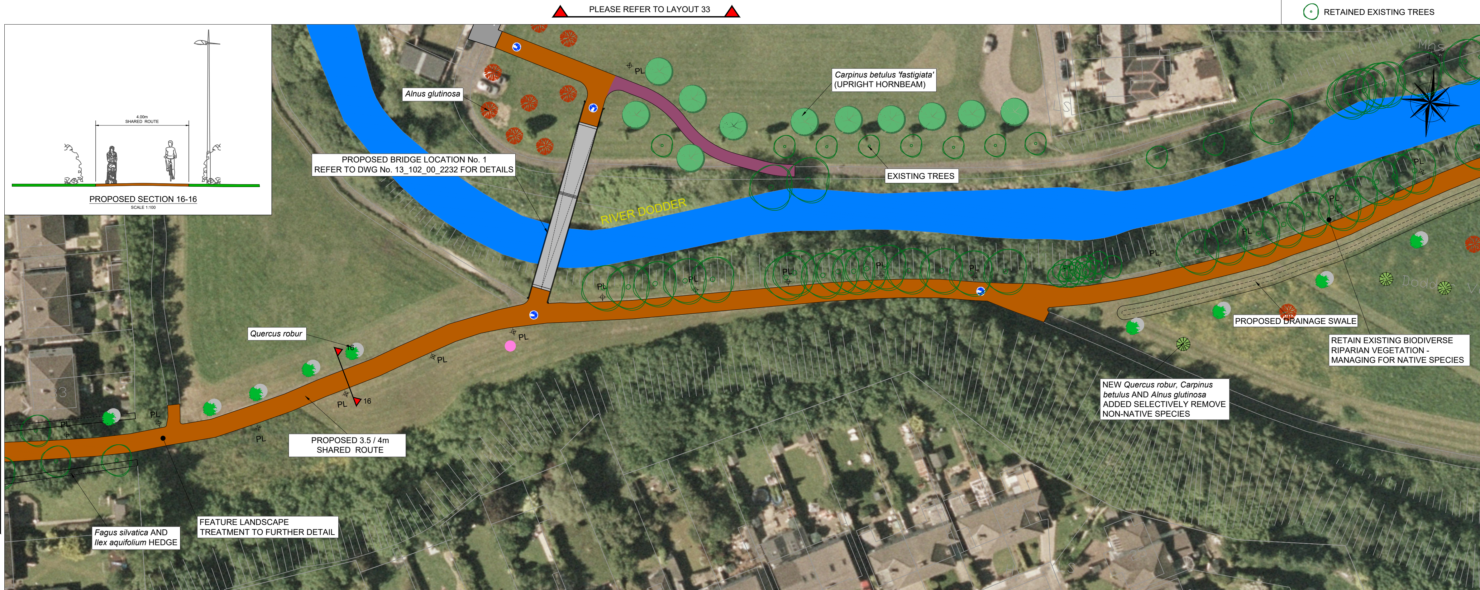
LAYOUT - 32 SCALE: 1:500
