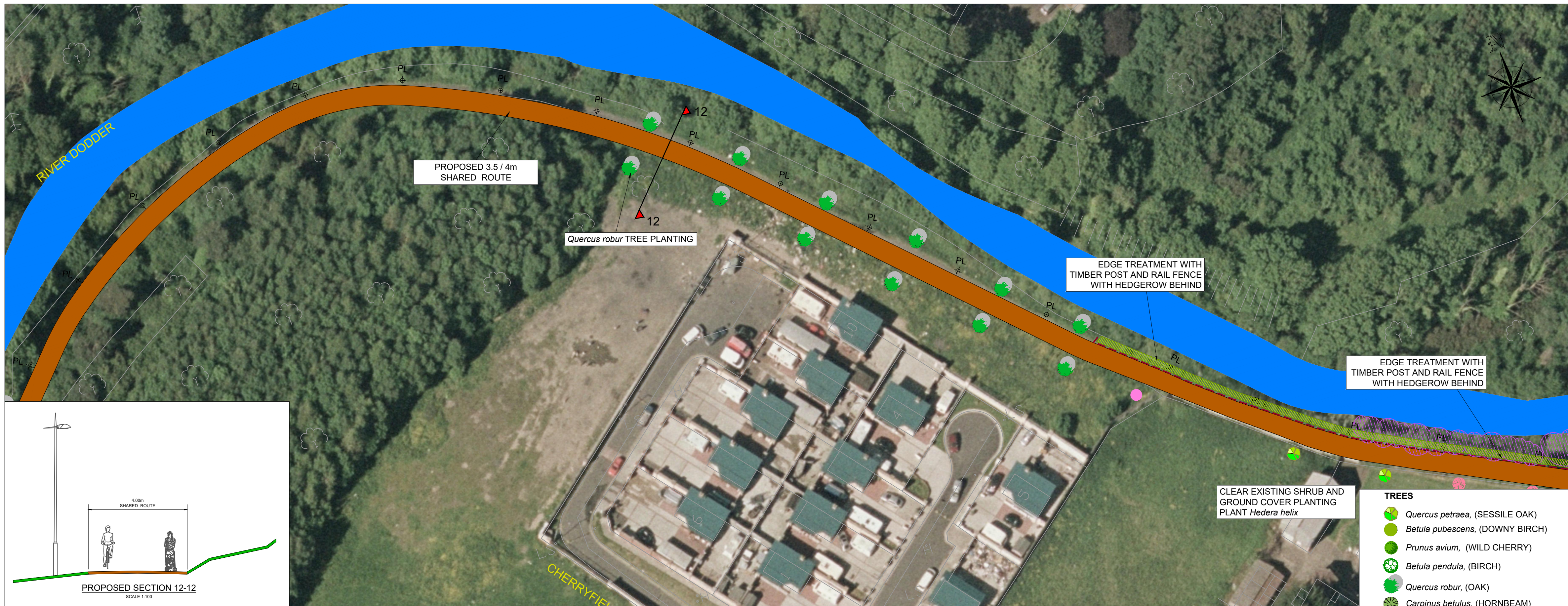
LAYOUT - 27 SCALE: 1:500
