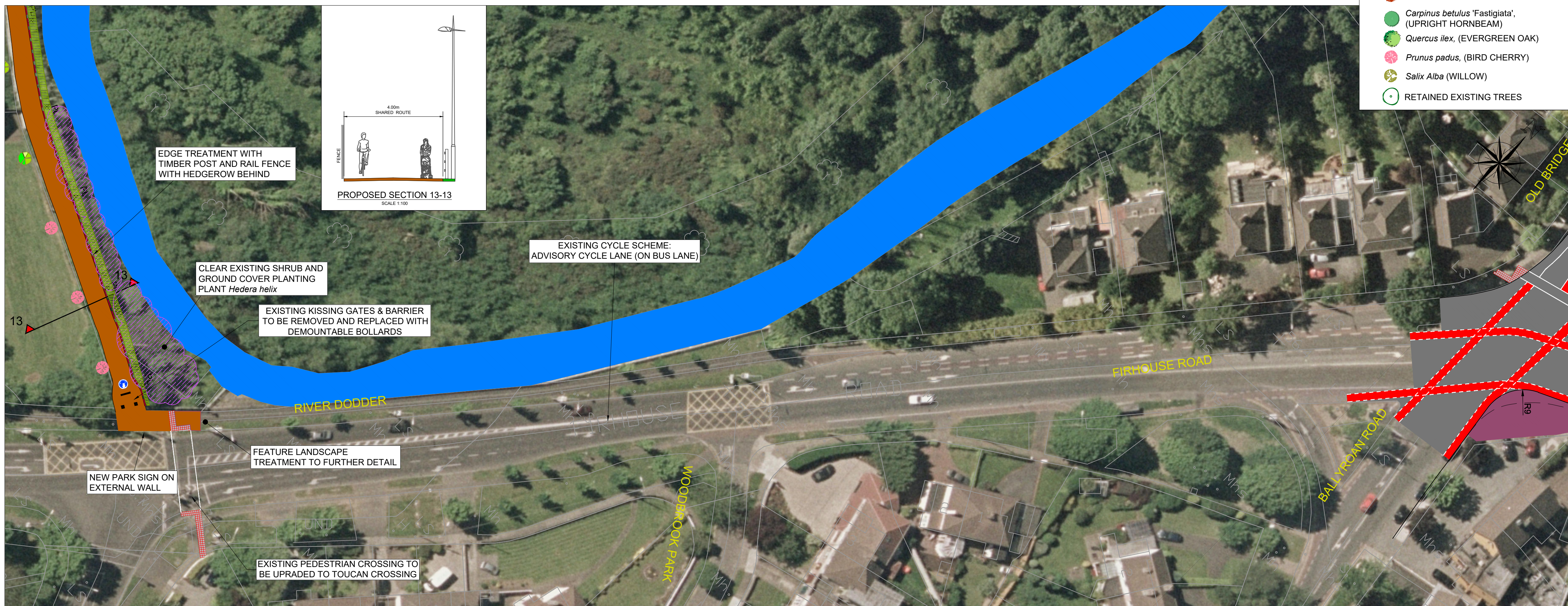
LAYOUT - 28 SCALE: 1:500
