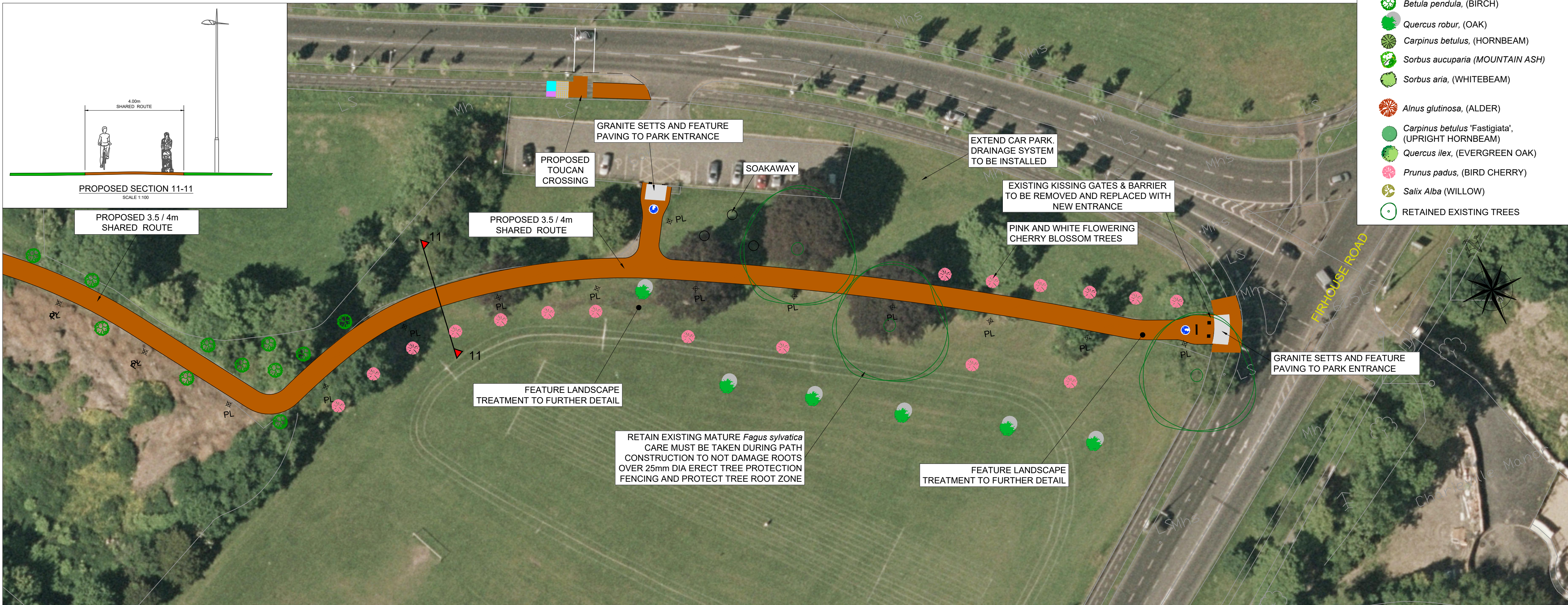
LAYOUT - 26 SCALE: 1:500
