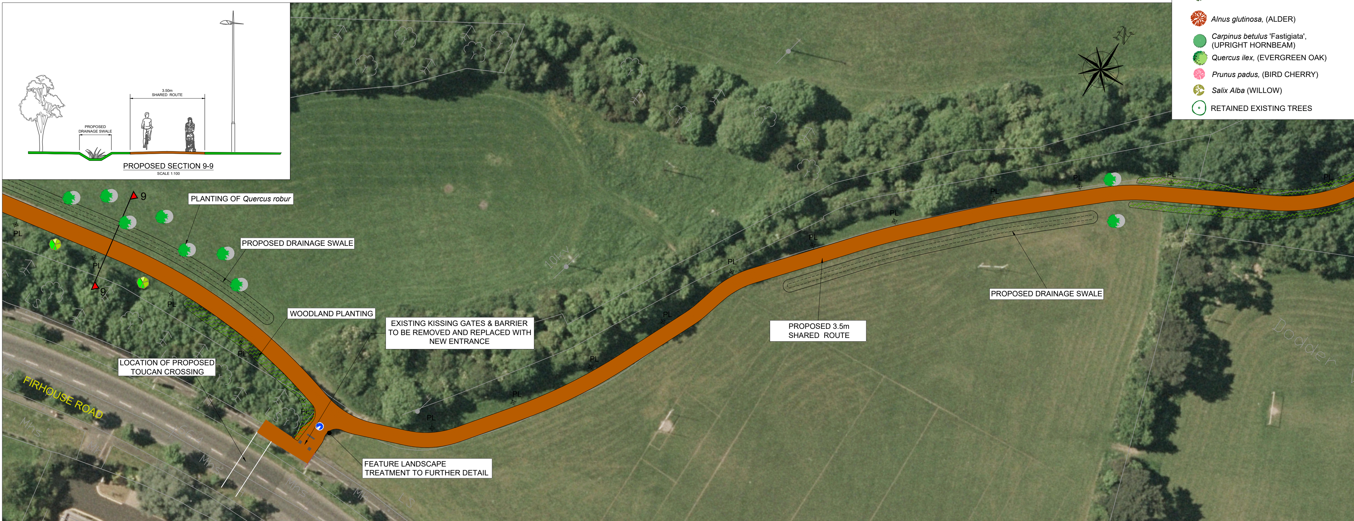
LAYOUT - 24 SCALE: 1:500
