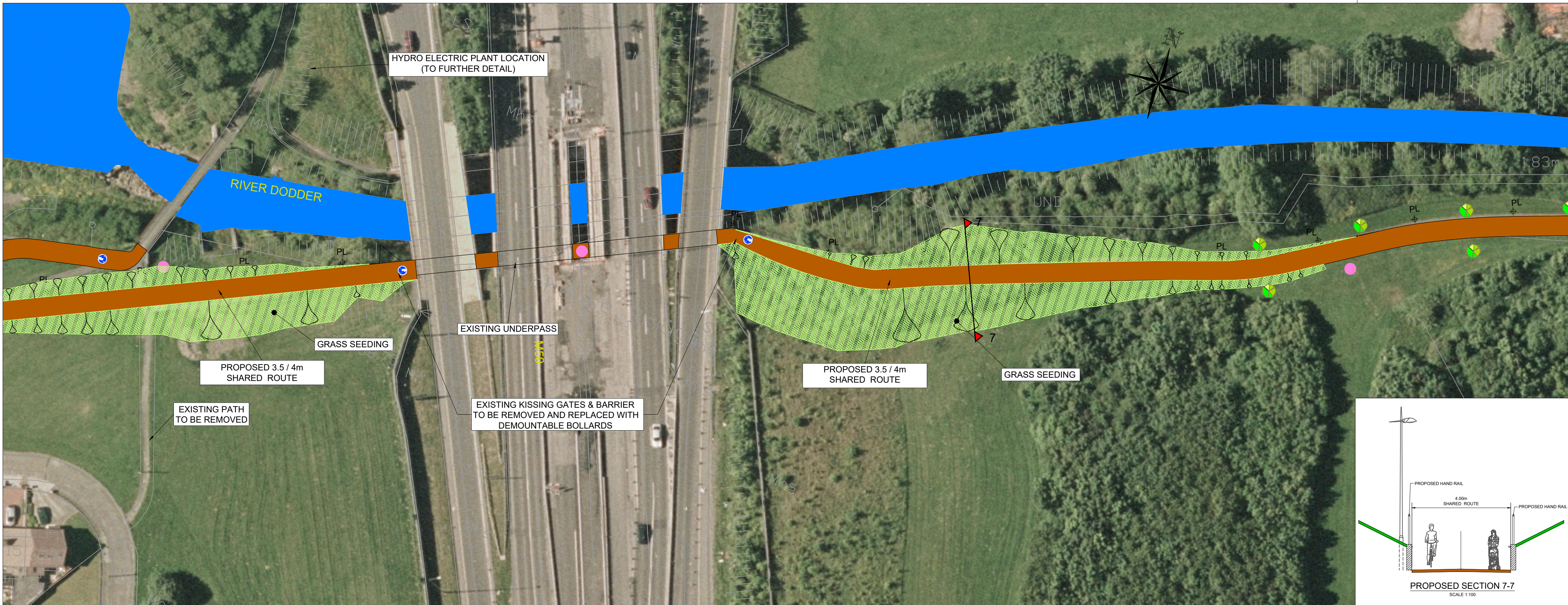
LAYOUT - 22 SCALE: 1:500
