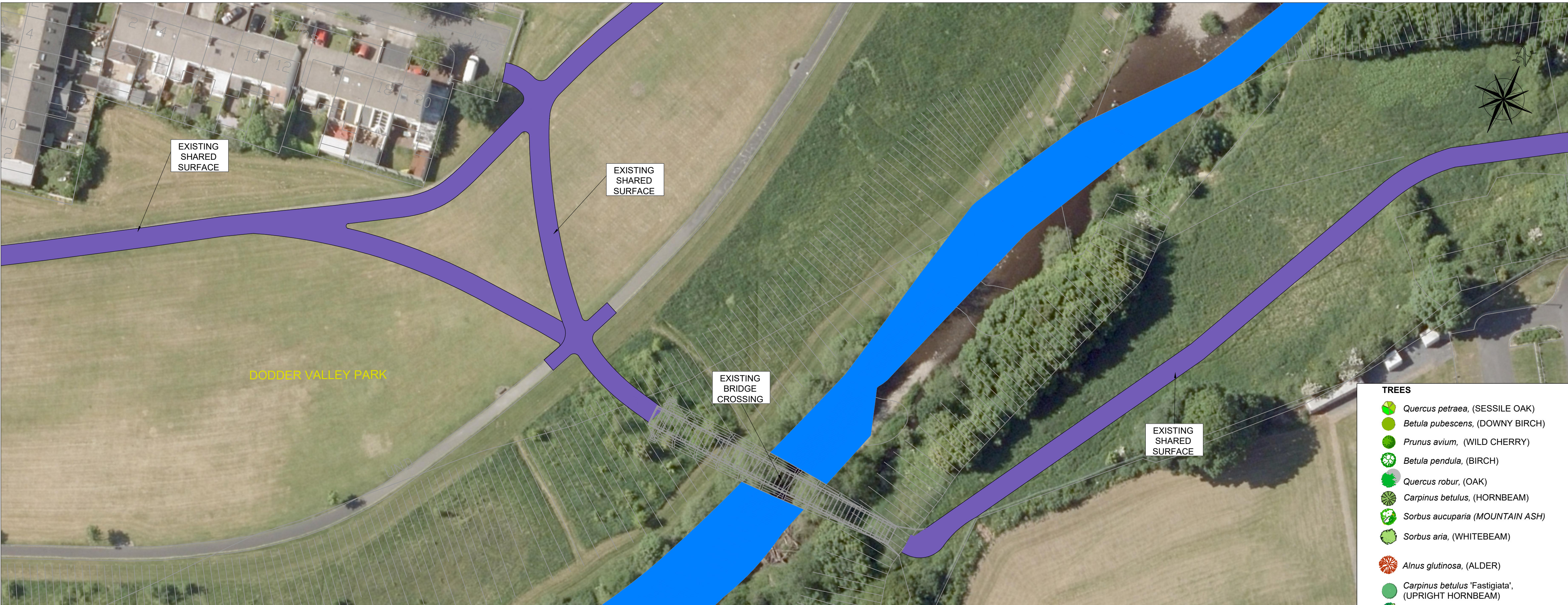
LAYOUT - 13 SCALE: 1:500
