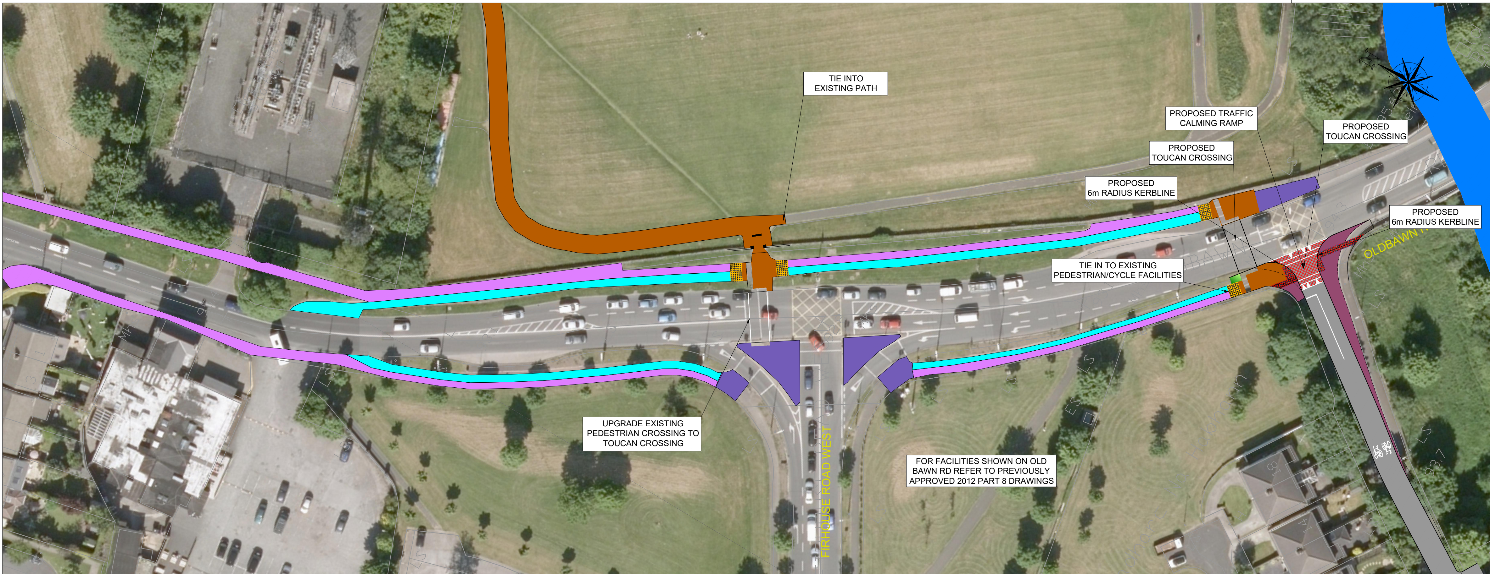
LAYOUT - 10 SCALE: 1:500
