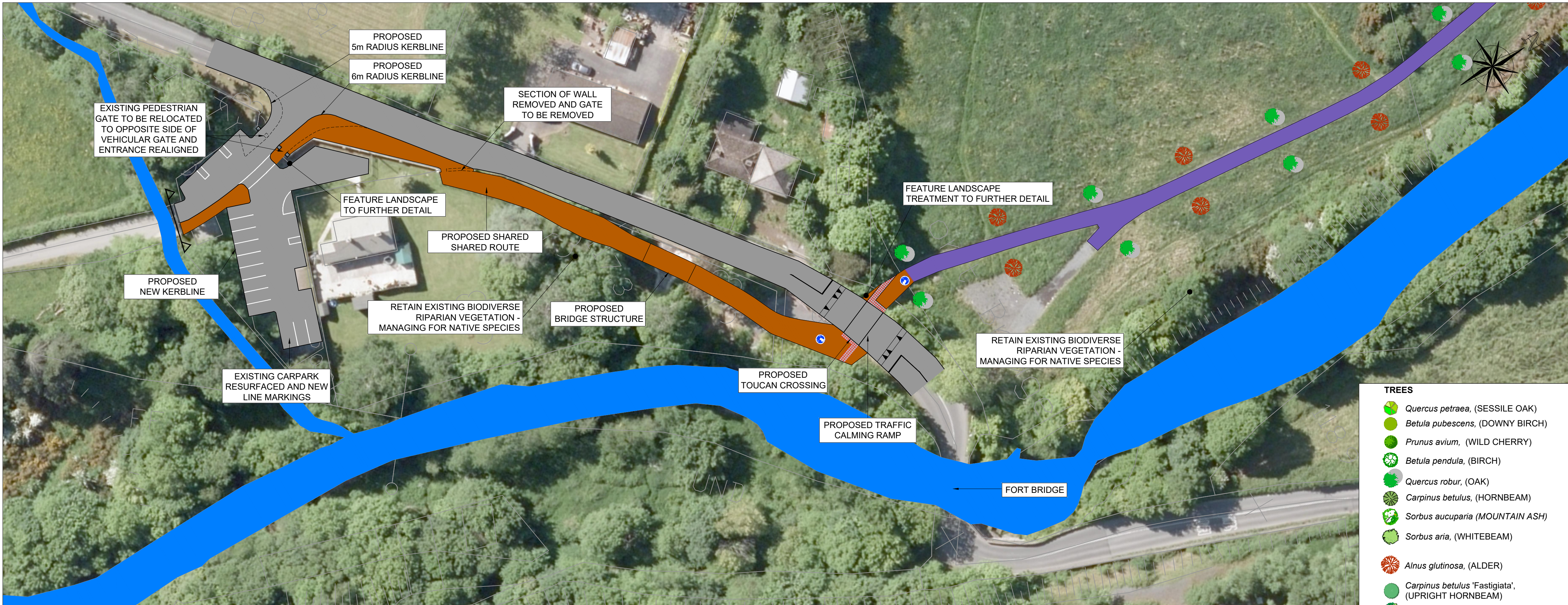
LAYOUT - 1 SCALE: 1:500
