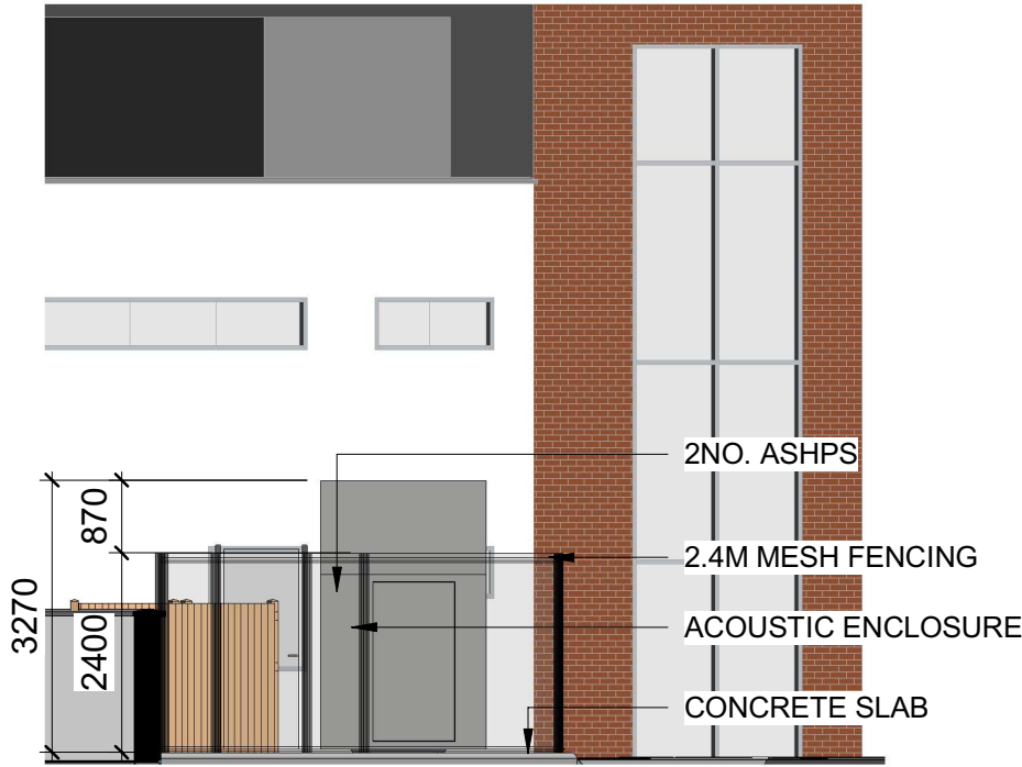
Section 2 1 : 100
