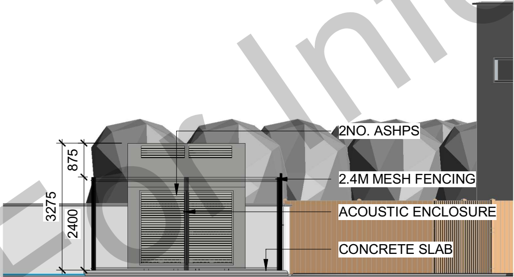
Section 1 1 : 100
