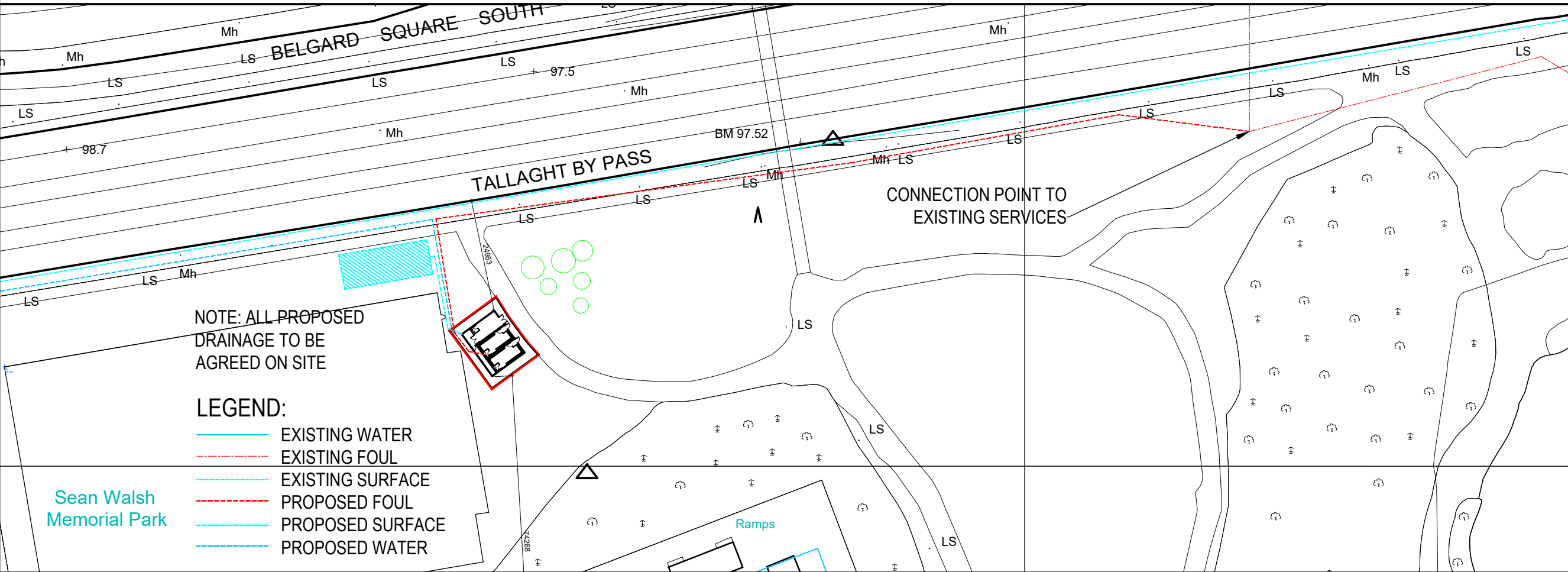
SITE PLAN DRAINAGE 1:1000
