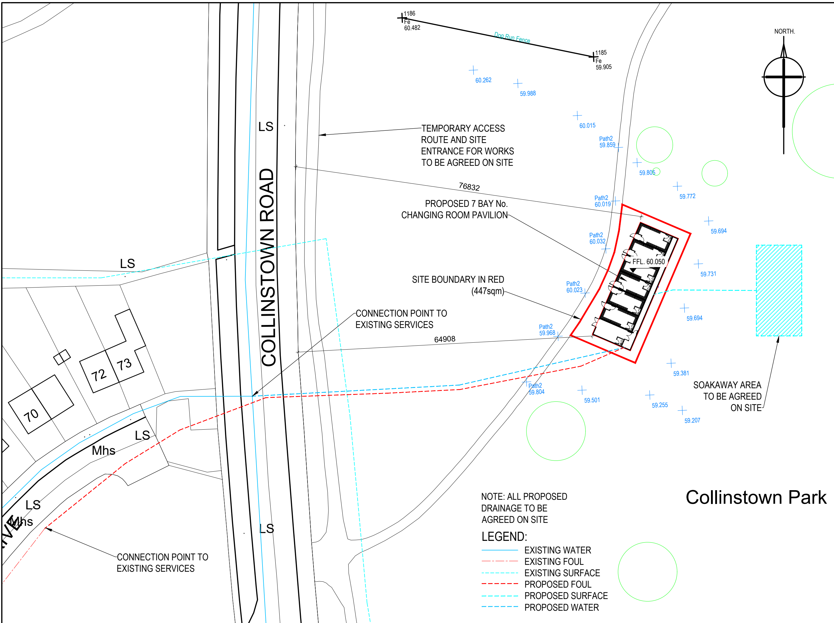
SITE PLAN 1:500
